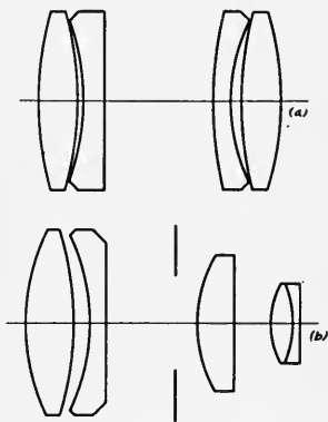
FIG. 4a. Kodak f/1.9 cine lens.
